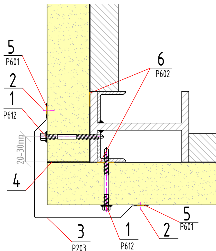
ŠIKMÝ ROHOVÝ PROFIL
